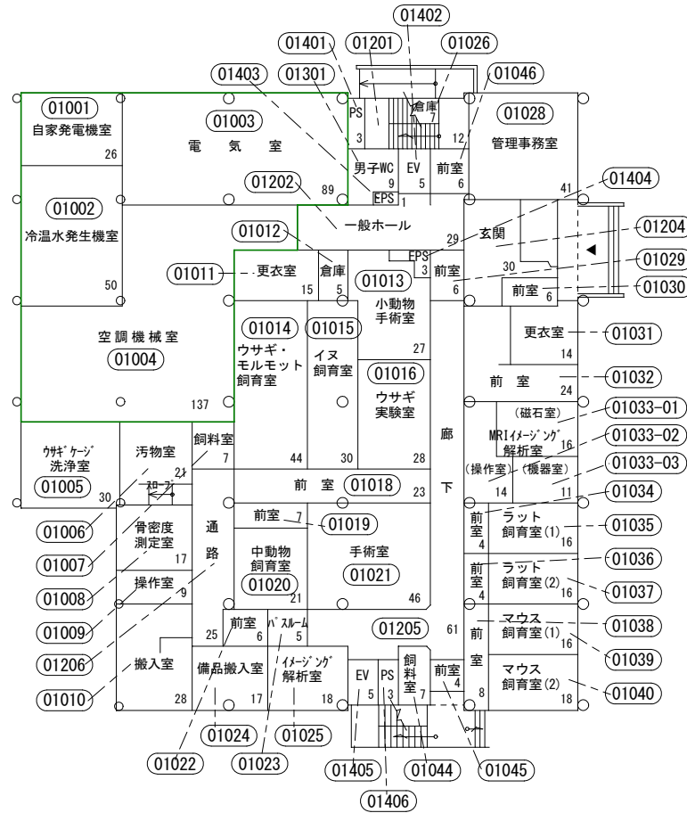
1階平面図 S = 1 / 400
