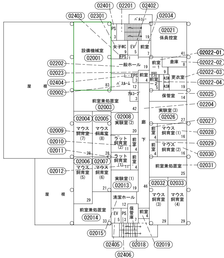
2階平面図 S = 1 / 4 0 0 (741㎡)
