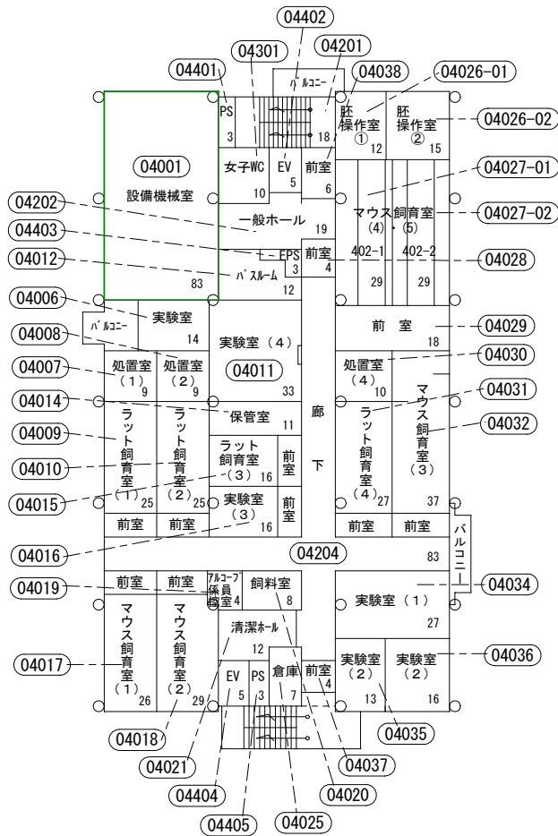
4階平面図 S = 1 / 4 0 0 (735㎡)
