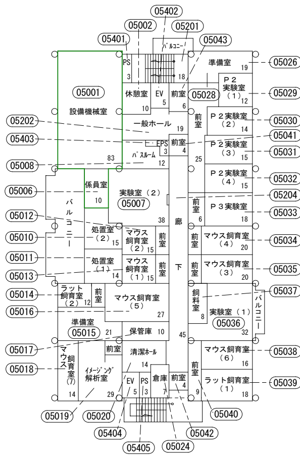
5階平面図 S = 1 / 4 0 0 (708㎡)
